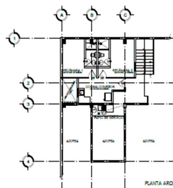
PLANTA ARQUITECTÓNICA ALTA RESIDENCIA MÉDICA
